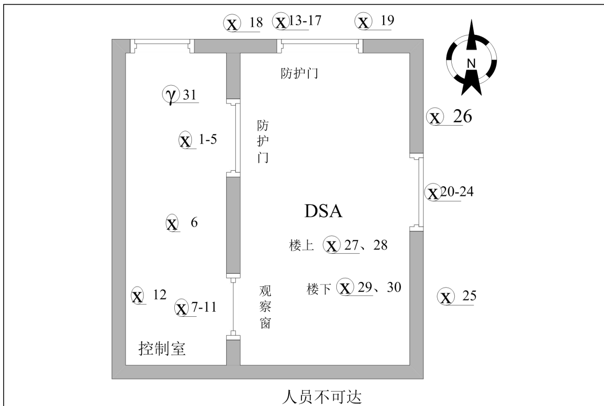
图 11-1 海安县人民医院西门子 Artis 型 DSA 验收监测点位示意图
