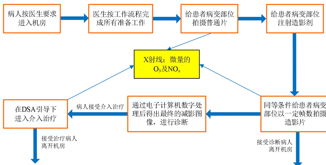
图 9-3 本项目 DSA 工作流程及产污环节示意图
