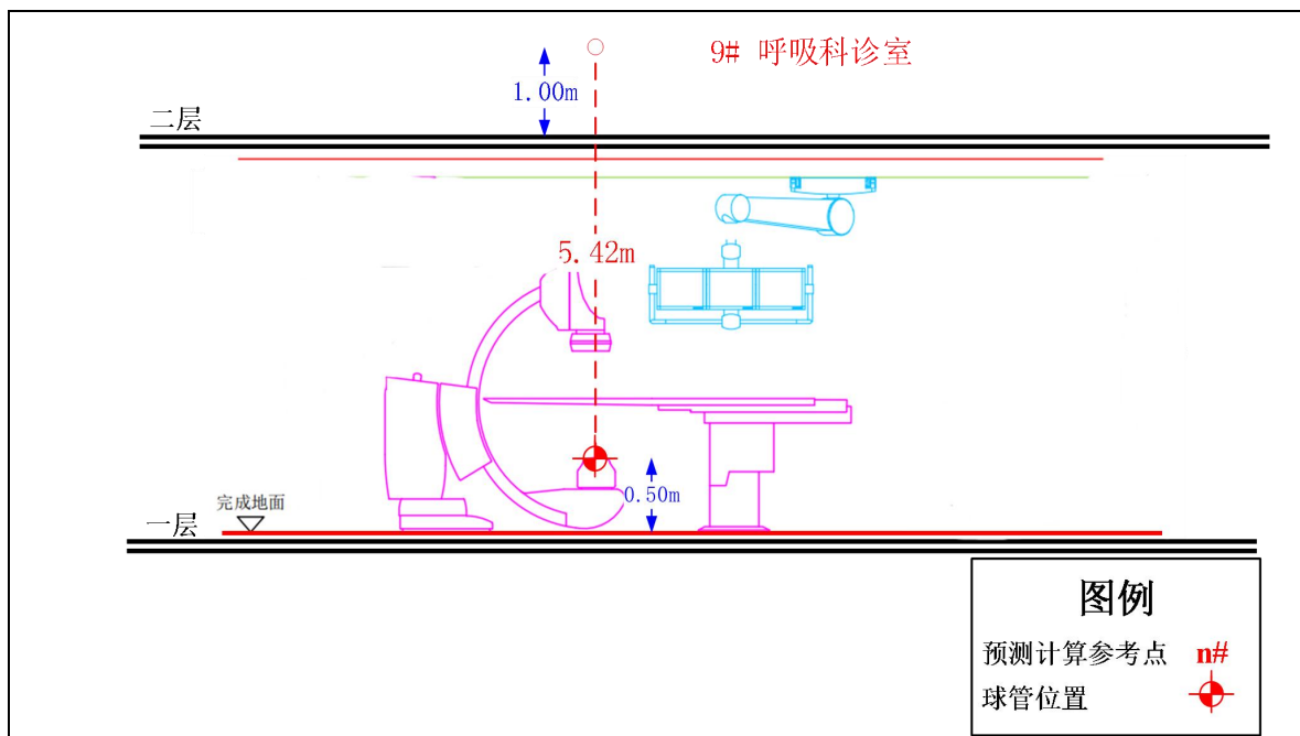
图 11-1 城西院区病房楼一楼介入室 DSA 机房检测点布设示意图
