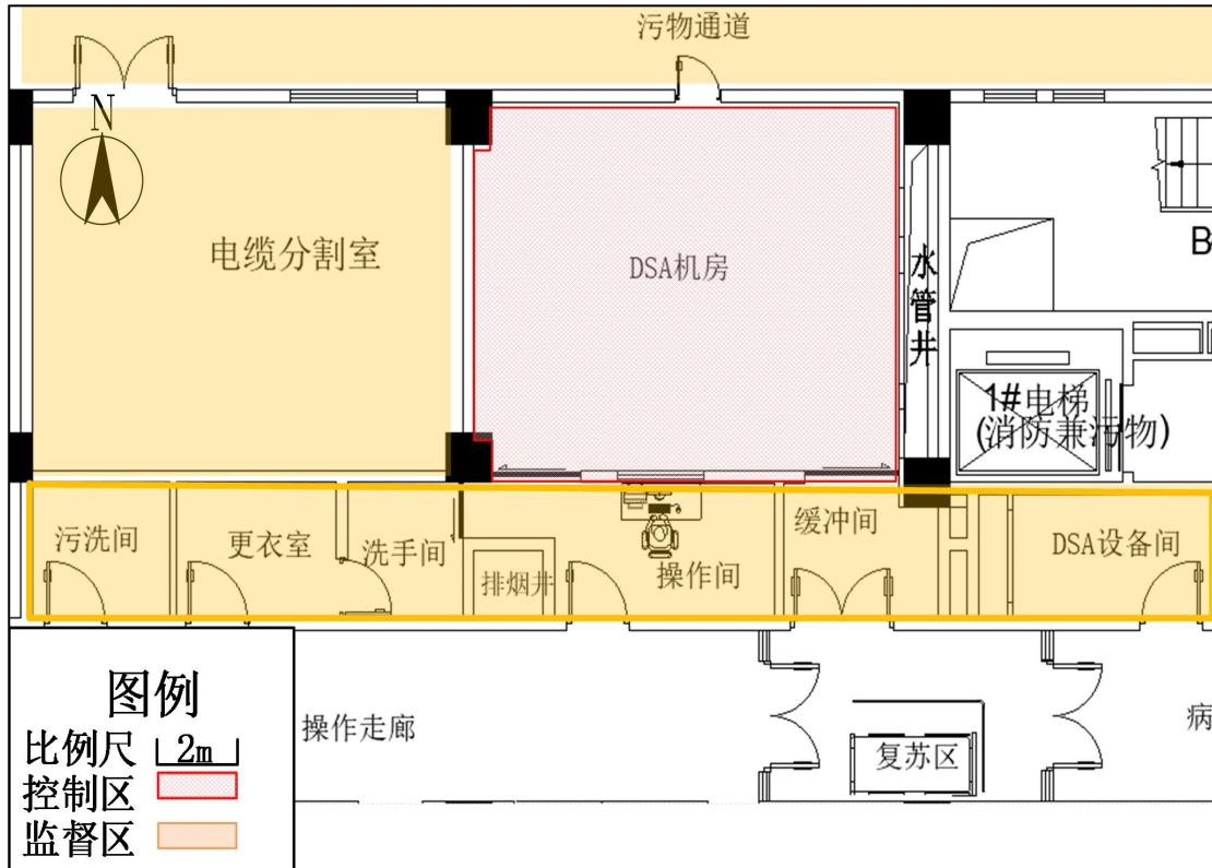
图 10-1 本项目 DSA 机房周围布置及分区示意图
