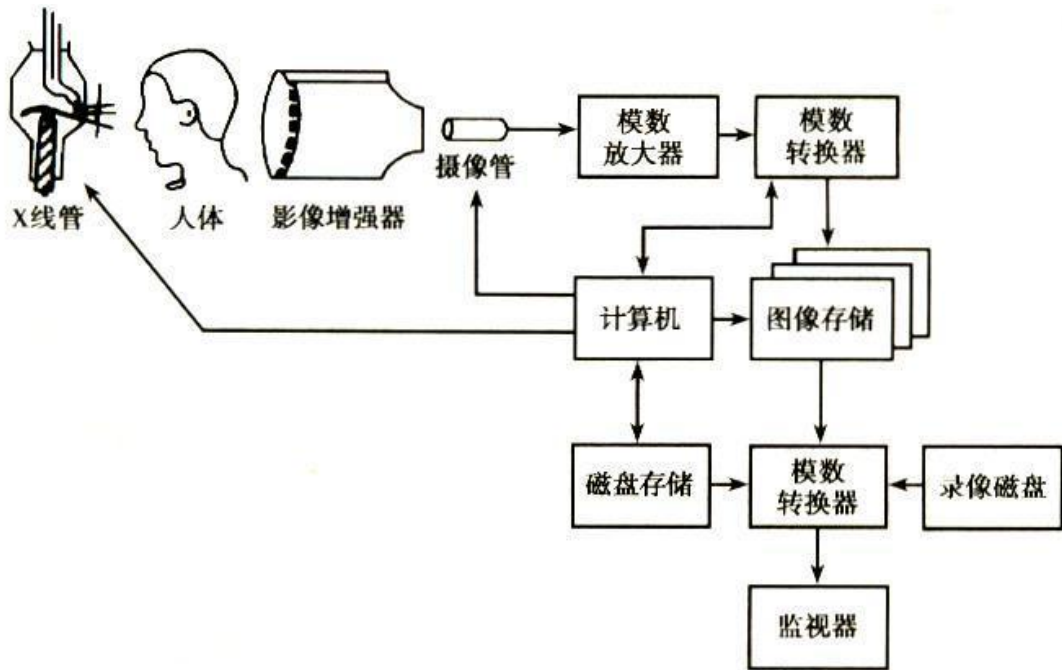
图 9-2 DSA 系统结构图
