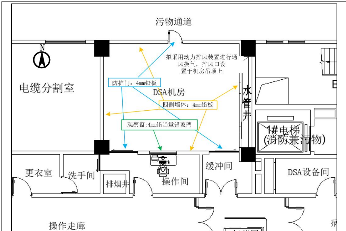
图 10-3 DSA 机房防护设计平面示意图
