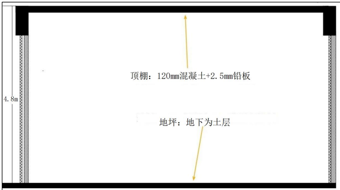
图 10-4 DSA 机房防护设计立面示意图
