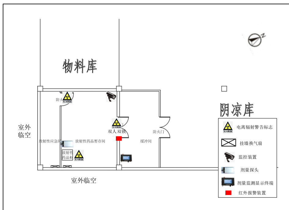
图 10-2 放射性药物暂存库辐射防护设施平面布置示意图
