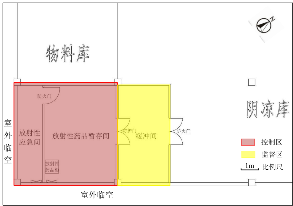
图 10-1 本项目放射性药物暂存库两区划分示意图
