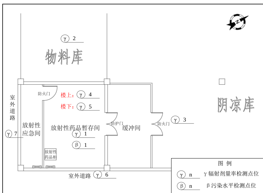
图 8-8 上药润天江苏医药有限公司新增暂存、销售放射性药物项目 拟建址周围 γ 辐射剂量率及 β 表面污染水平监测点位示意图
